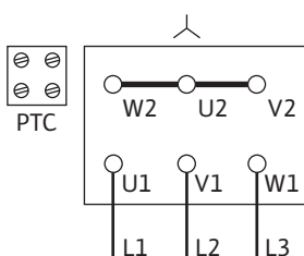
Fig. 14: Переключение Y
