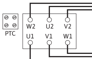
Fig. 15: Переключение Y-Δ
