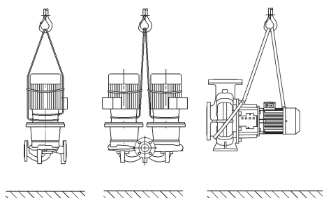
Fig. 1: Транспортировка насоса
