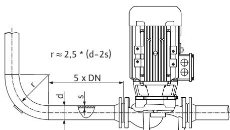
Fig. 12: Участок выравнивания потока перед и за насосом
