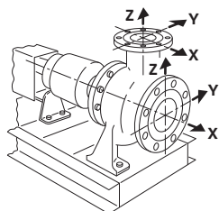
Fig. 8: Случай нагрузки 1A
