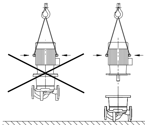
Fig. 2: Транспортировка электродвигателя
