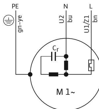
Fig. 6: Схема подсоединения 1~ электродвигателя
