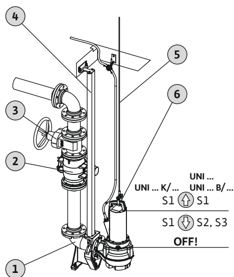
Fig. 5: Стационарная установка в погруженном состоянии
