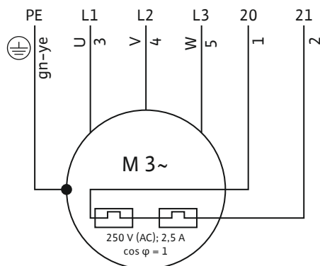
Fig. 8: Схема подсоединения 3~ электродвигателя
